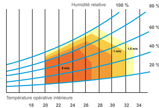
Le diagramme de Givoni
